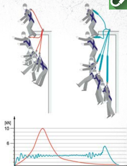
Slika 1. Poređenje apsorber energije i uže
